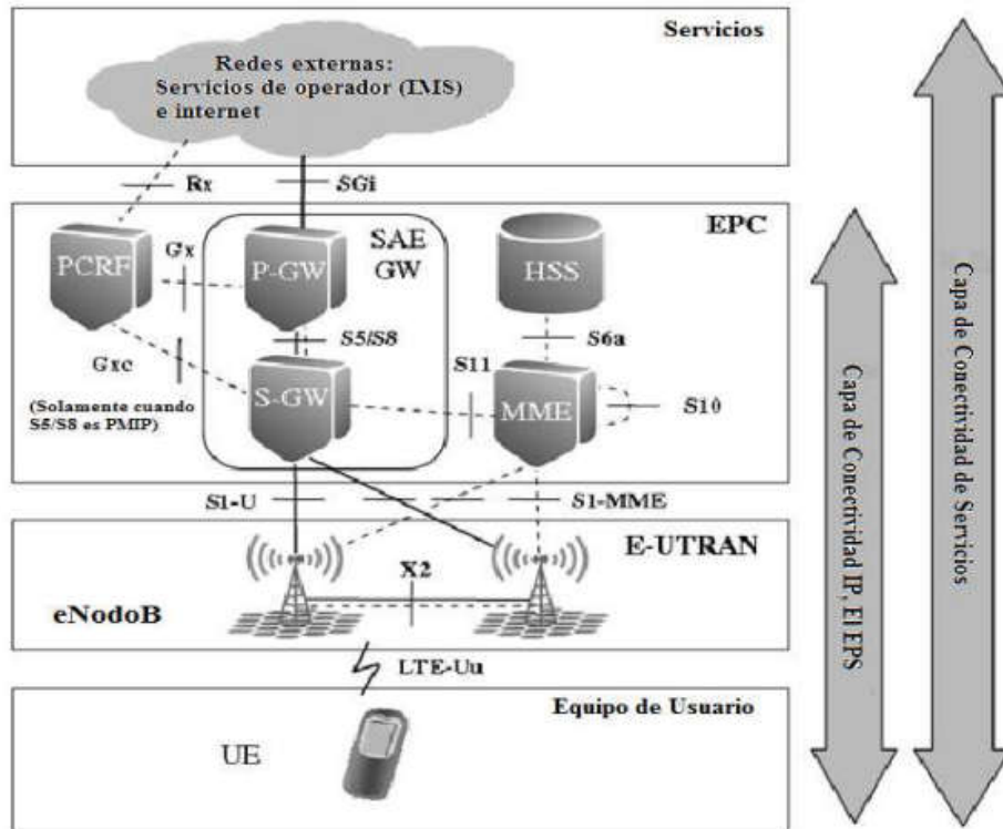
Figura 1. Arquitectura de la red 4G
