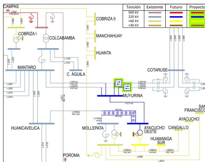
Figura N° 1: Esquema unifilar de los Equipos FACTS Serie de LT 220 kV Muvurina-Cotaruse en SE Muvurina.
