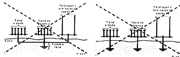
Figura 3. Puestas a tierra separadas o independientes
