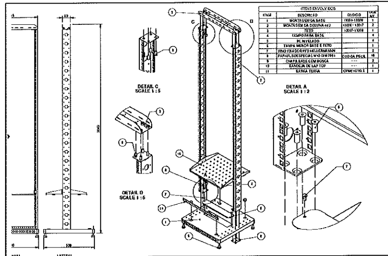
Esquema de Rack de Comunicaciones
