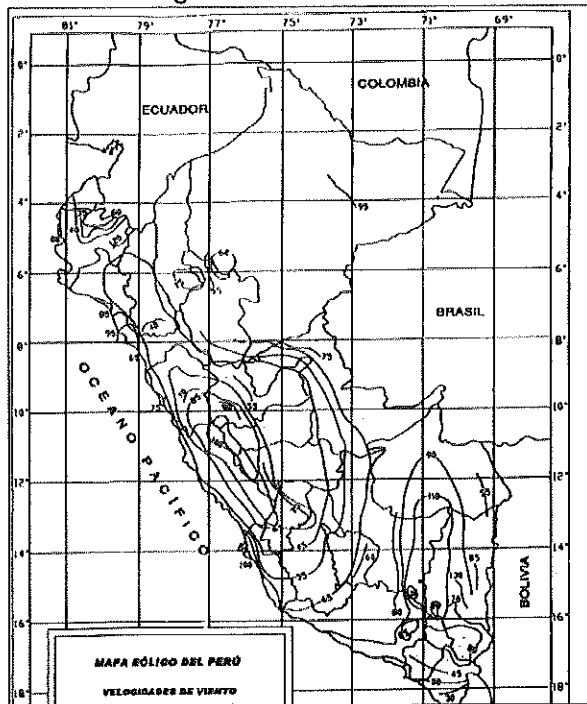
Mapa Eólico para determinar velocidades de viento (Fuente Norma E.020)
