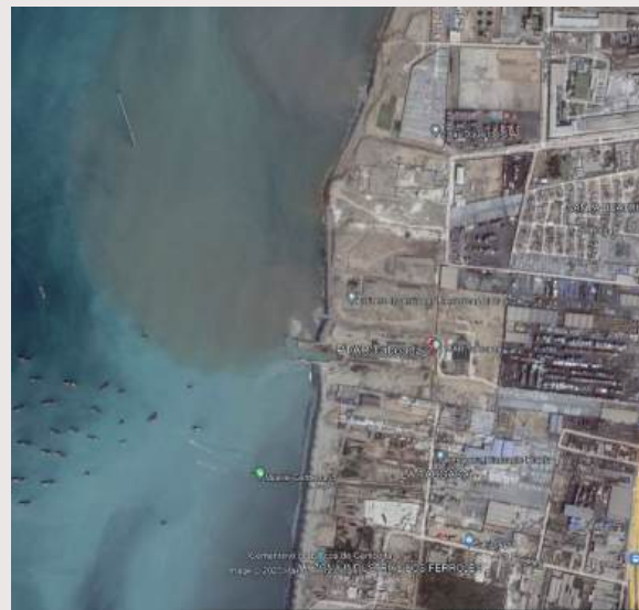
Ilustración 18: Área PTAR Taboada II semestre de 2012
