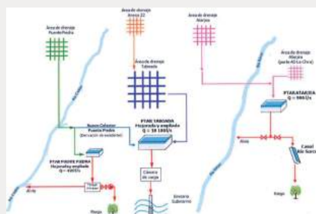
ILUSTRACIÓN 21 Diagrama de tratamiento zona centro-norte
