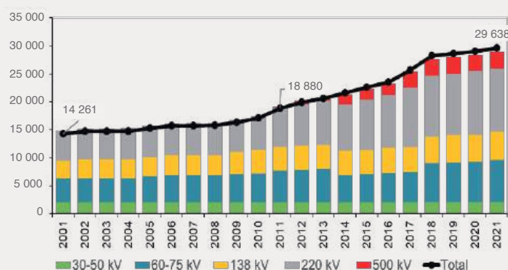
Ilustración 17 Evolución de las líneas de transmisión en el Perú
